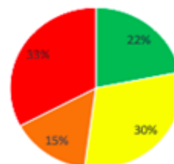
Cílová destinace vystěhovalectví - generace 35 let+, n=119
