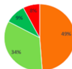
Vystěhovalecké tendence - generace 35 let a starší, n=211
