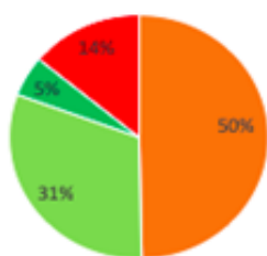
Vystěhovalecké tendence - generace mileniánů, n=300
