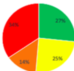
Cílová destinace vystěhovalectví - mileniáni n=191
